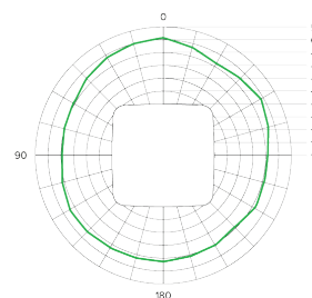
A42 5 GHz
