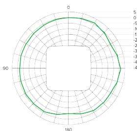
A42 2.4 GHz
